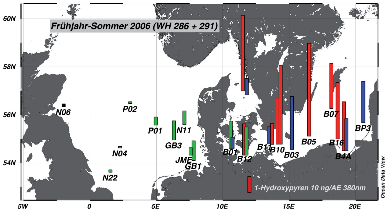
Abb. 5: 1-Hydroxypyren [ng/AE 380nm] in Fischen; Mittelwerte von je ca. 20 Tieren aus Frühjahr und Sommer 2006: Klieschen (grün), Flundern (rot) und Dorsch (blau). Die Ostsee-Werte sind zum Vergleich mit abgebildet
